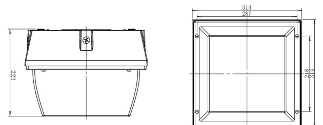
60w Dimensions
