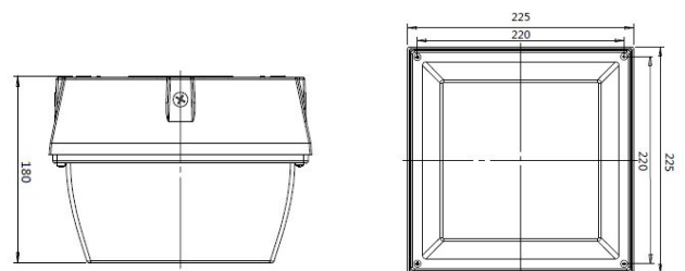
40w Dimensions
